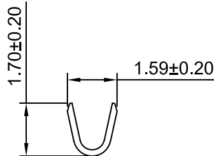
SEC: B-B
