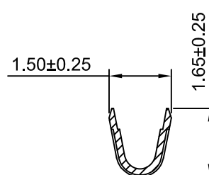
SEC:B-B
