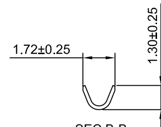
SEC:B-B
