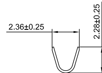
SEC:A-A
