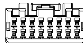
2x8P Type 1
