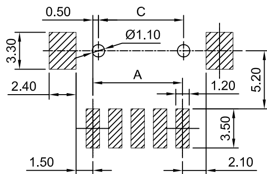
P.C.B LAYOUT 4P~15P
