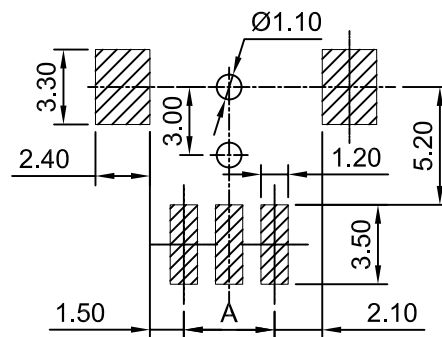
P.C.B LAYOUT 2P~3P
