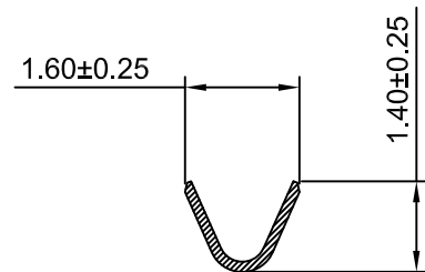
SEC:B-B
