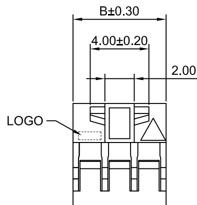
2x3P~2x25P
