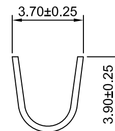
SEC:A-A
