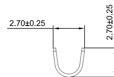
SEC:A-A
