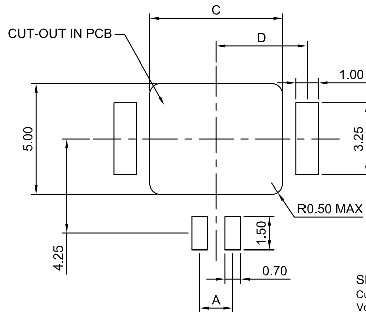
P.C.B LAYOUT
