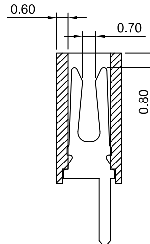
SEC: A-A
