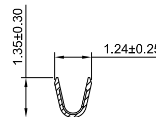
SEC: B-B
