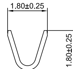
SEC:A-A
