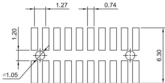
P.C.B LAYOUT
