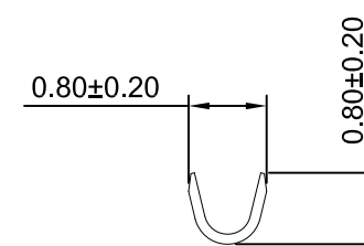
SEC: B-B
