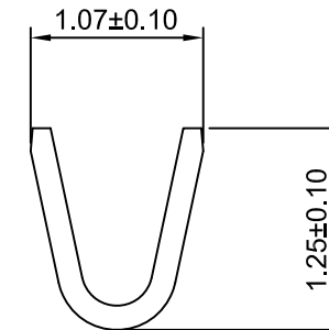
SEC: A-A
