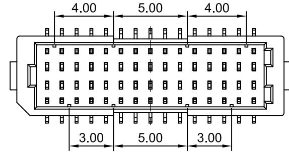
2x15P
