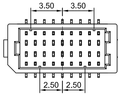
2x9P
