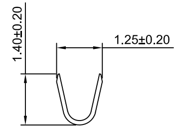
SEC:A-A
