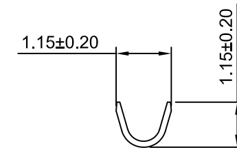
SEC:B-B
