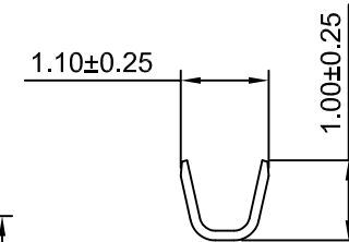
SEC: A-A
