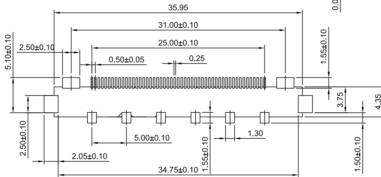
P.C.B LAYOUT
