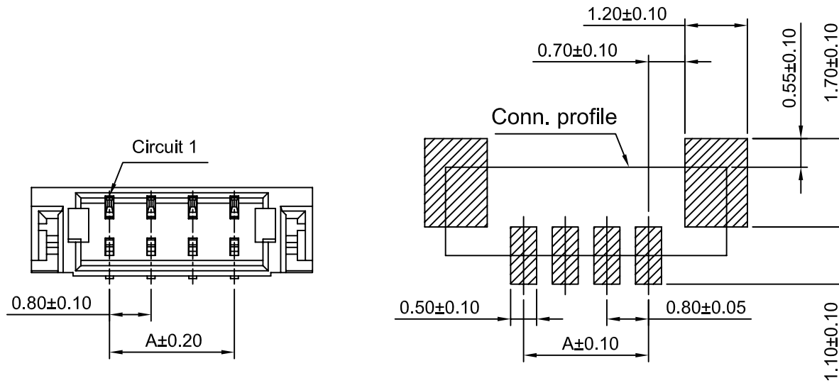
P.C.B. LAYOUT
