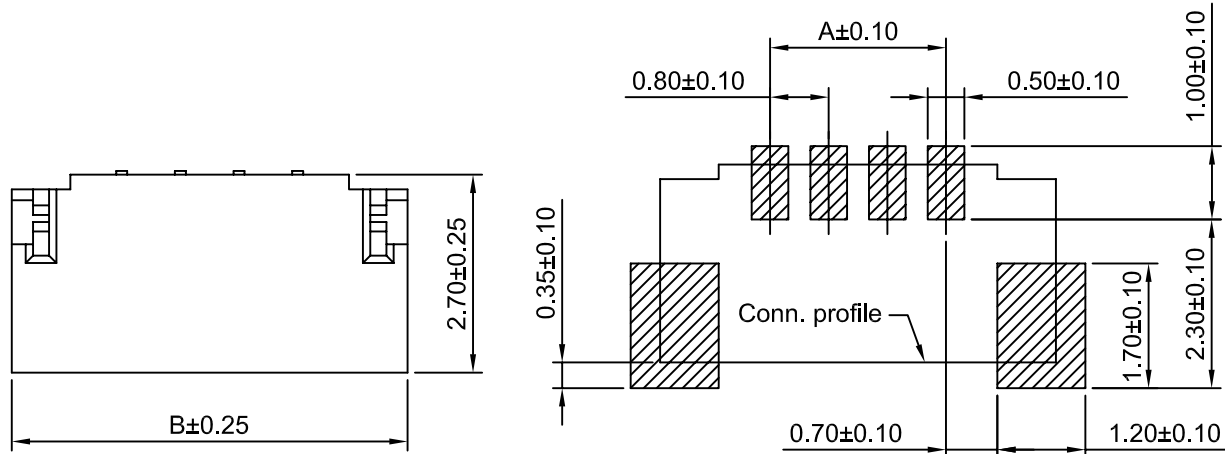
P.C.B. LAYOUT
