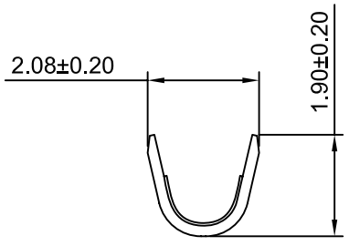
SEC:B-B
