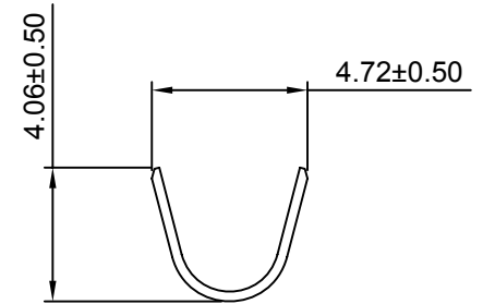
SEC:A-A
