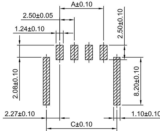
P.C.B LAYOUT
